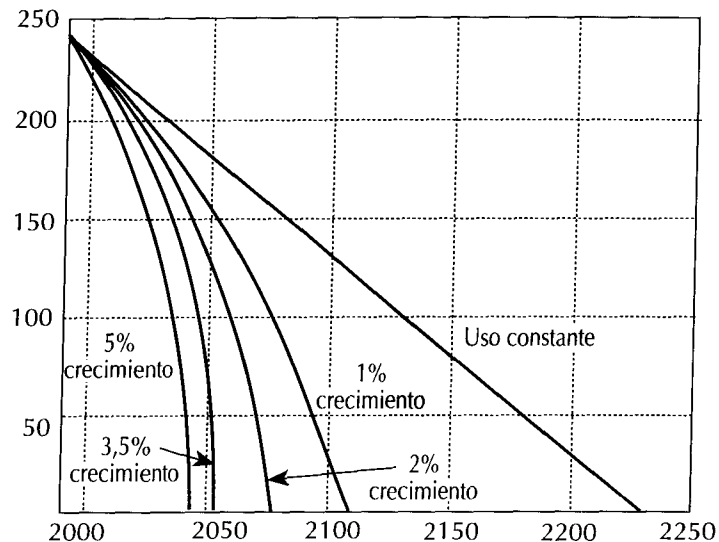
Ilustración 3-11 AGOTAMIENTO DE LAS RESERVAS MUNDIALES DE GAS SUPONIENDO DIFERENTES TASAS DE CRECIMIENTO EN EL CONSUMO
