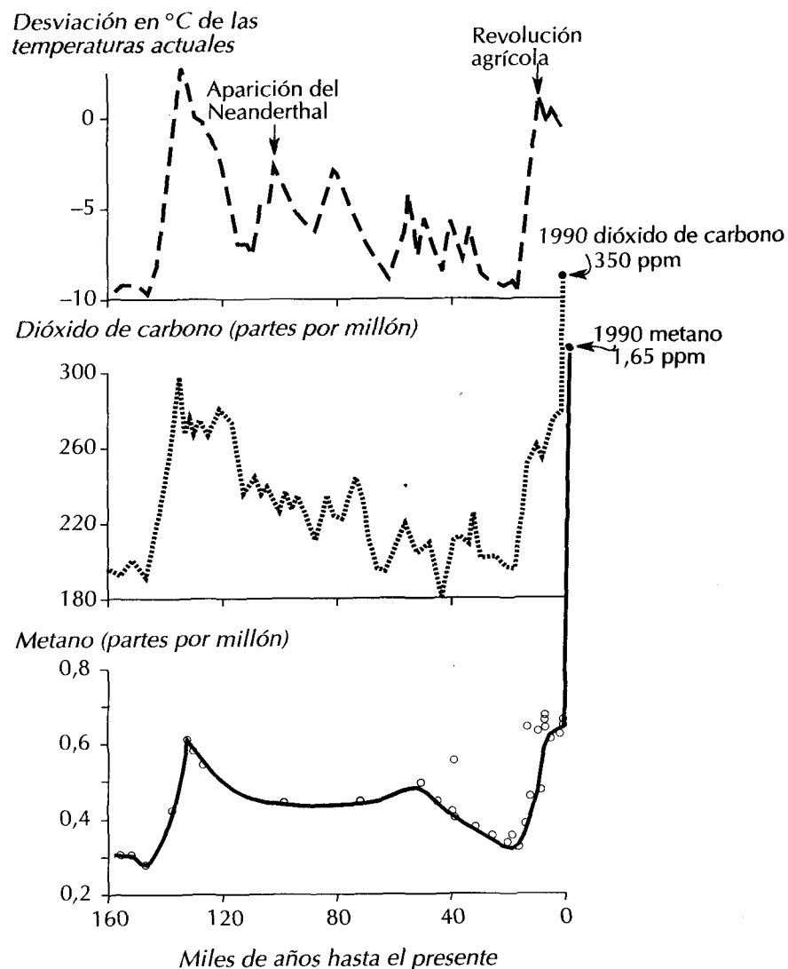
Ilustración 3-23 GASES DE INVERNADERO Y TEMPERATURA GLOBAL DURANTE LOS ÚLTIMOS 160.000 AÑOS
