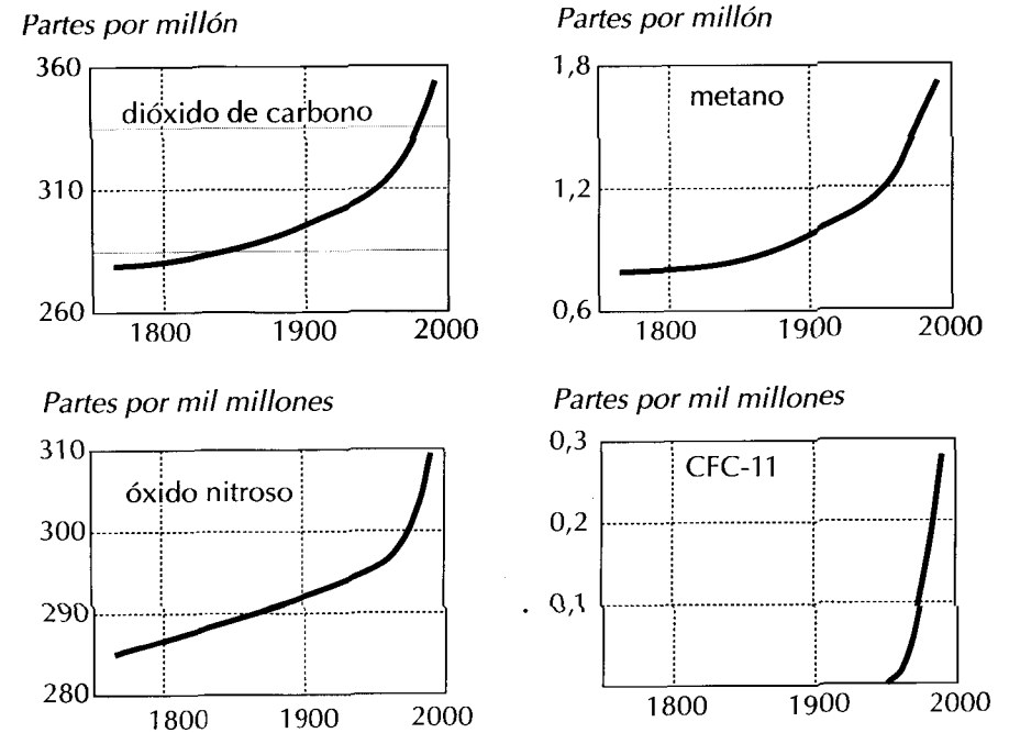
Figura 3-21 CONCENTRACIONES GLOBALES DE GASES DE EFECTO INVERNADERO
