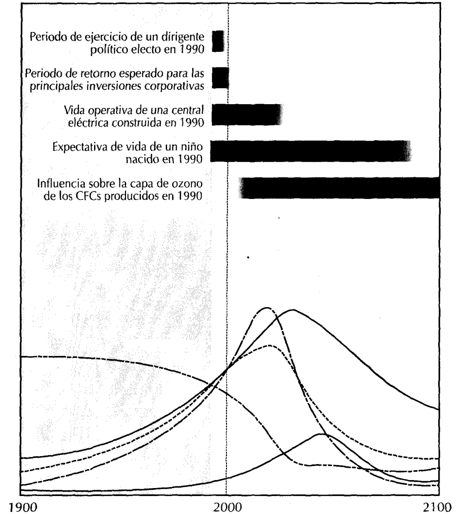
Ilustración 8-1 HORIZONTE TEMPORAL DEL MODELO WORLD3
