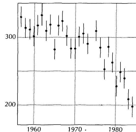
Ilustración 5-4 MEDICIÓN DEL OZONO EN BAHÍA HALLEY, ANTÁRTIDA
