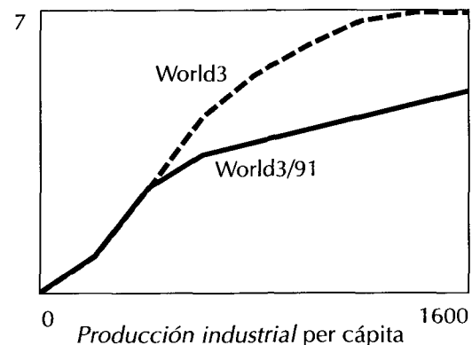
Ilustración A-14 GRÁFICO REVISADO DE LA RELACIÓN ENTRE PRODUCCIÓN INDUSTRIAL Y UTILIZACIÓN PER CÁPITA DE RECURSOS NO RENOVABLES
