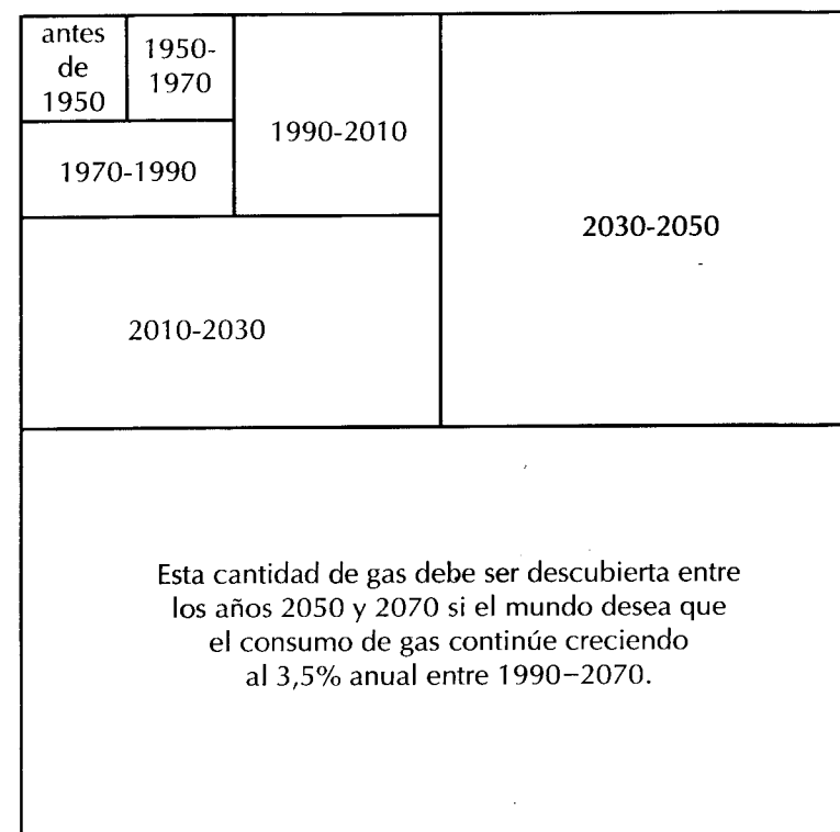
Ilustración 3-12 DESCUBRIMIENTOS NECESARIOS DE GAS PARA MANTENER UNA TASA DE CRECIMIENTO ANUAL DEL 3,5%
